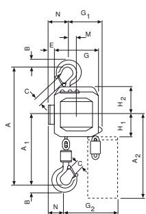
Модель CPE/CPEF на крюке, 1.600 - 3.000 кг, одноветвевая
