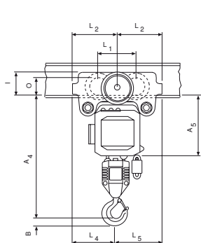
Модель CPE/CPEF на крантележке без привода или с мех. приводом
