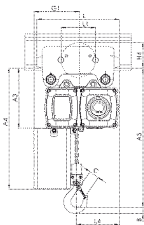
Модель CPV/CPVF на крантележке с мех. приводом
