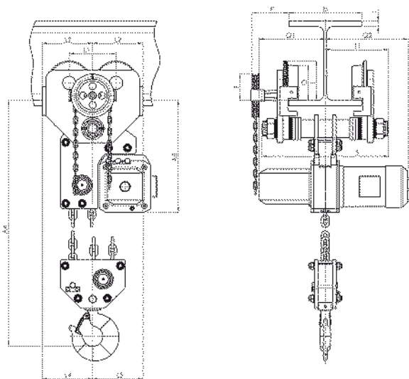
Модель CPE/CPEF на крантележке с мех. приводом, 7.500 кг
